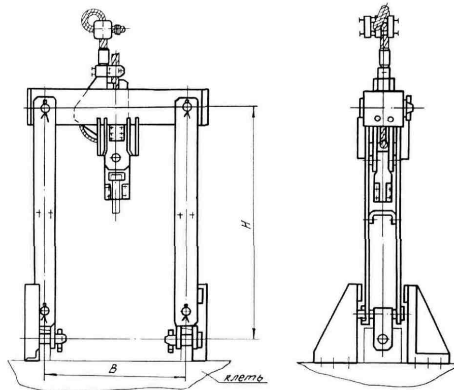
Основные параметры и размеры подвесных устройств УП для шахтных клеток
